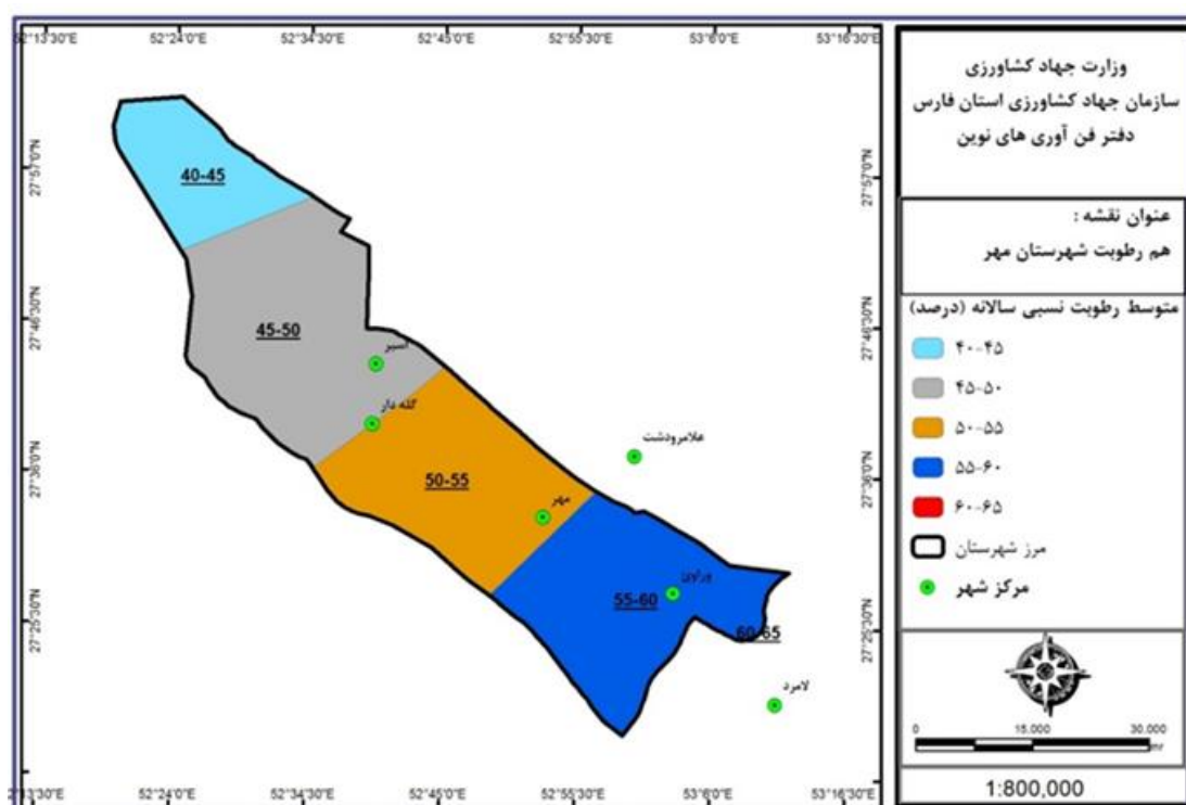
شکل ۵. نقشه هم رطوبت شهرستان مهر
