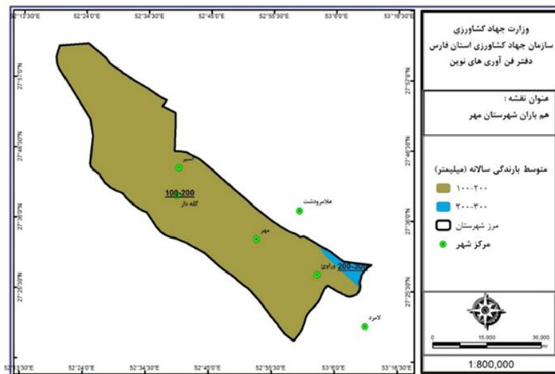
شکل ۴. نقشه هم باران شهرستان مهر
