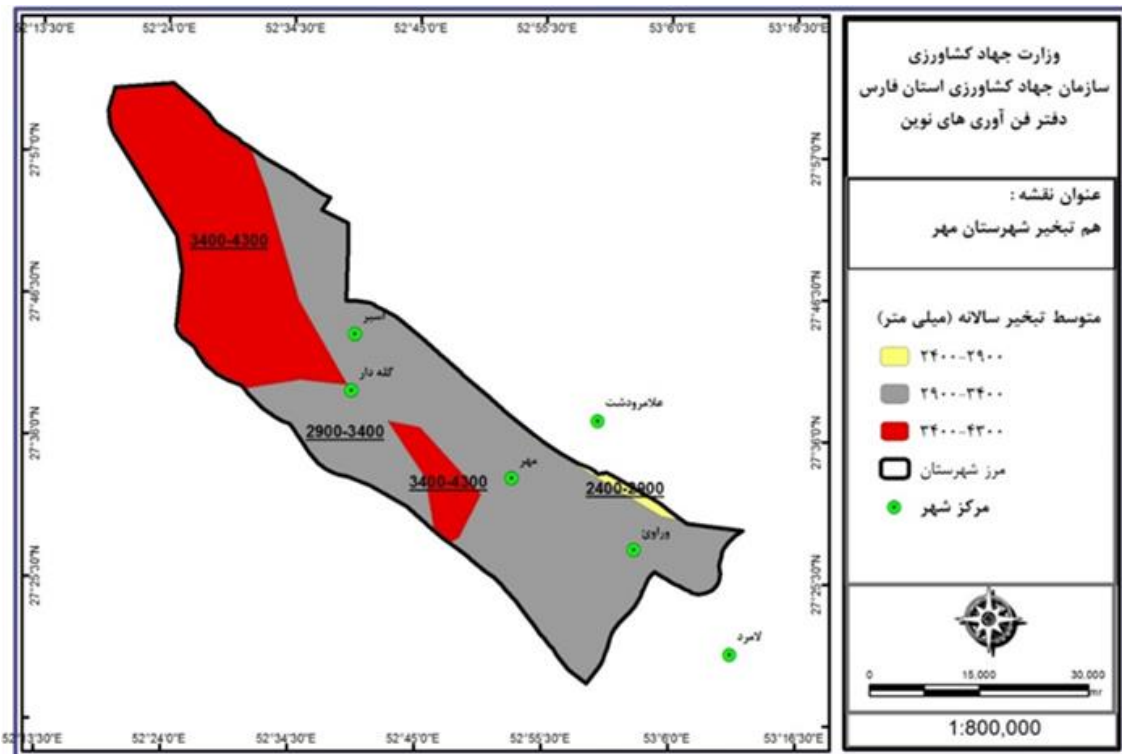
شکل ۶. نقشه هم تبخیر شهرستان مهر
