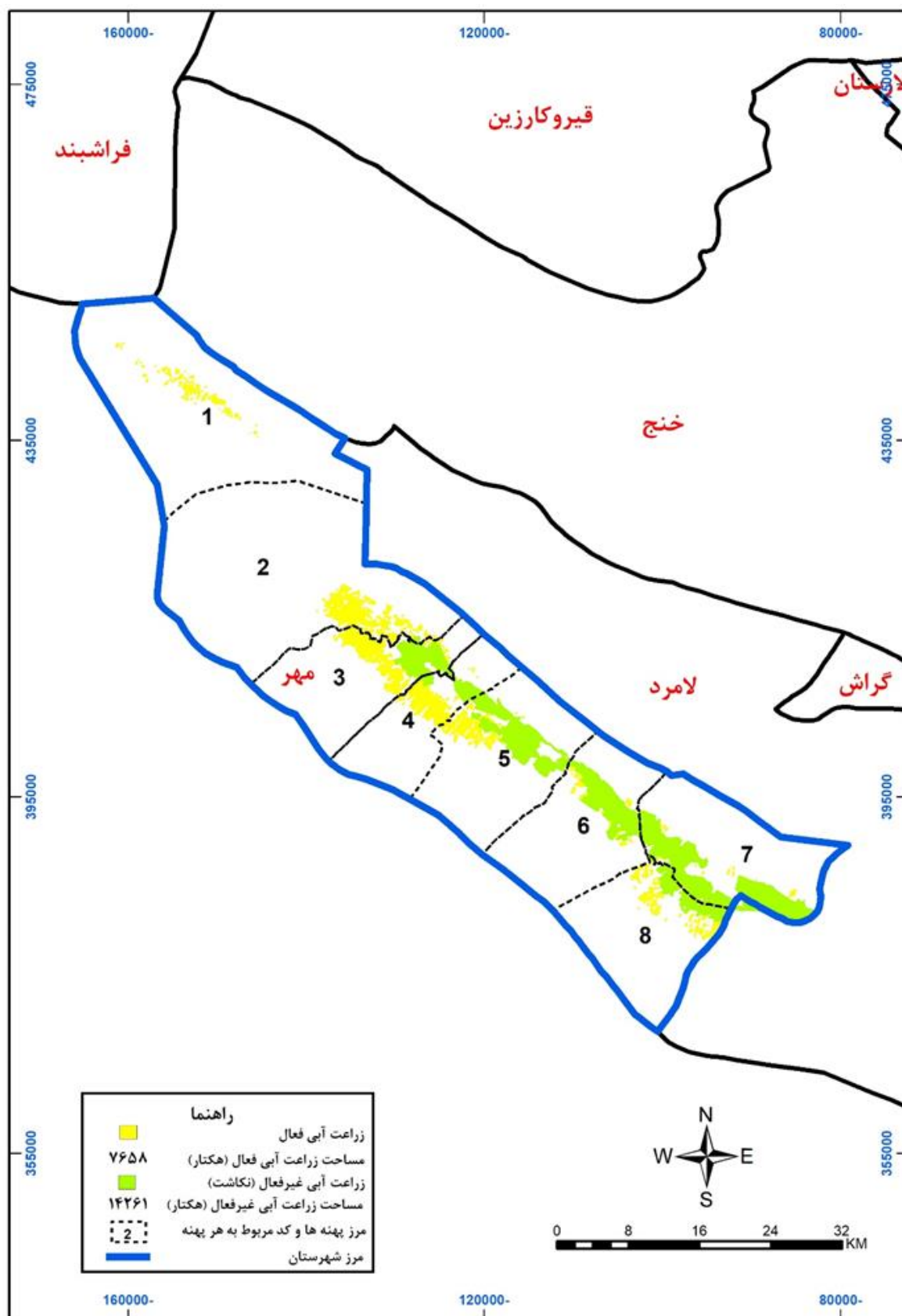
شکل 10. نقشه پراکنش زراعت آبی سال ۹۸-۱۳۹۷ شهرستان مهر
