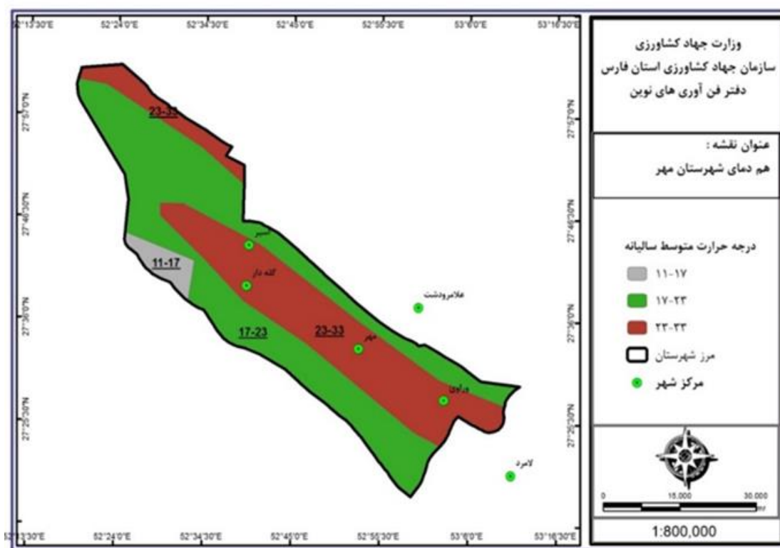
شکل ۳. نقشه هم دمای شهرستان مهر
